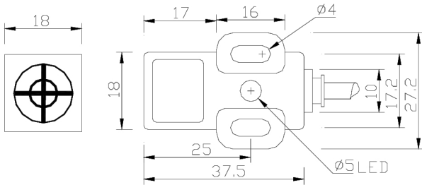
導線引出型
